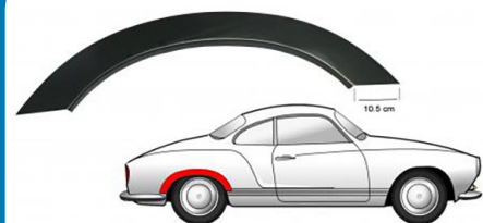
Tôle de réparation pour joue d'aile arrière droite ou gauche (la pièce) Ghia
