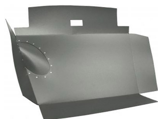
Carton de coffre avant Ghia de 8.1967 et après
