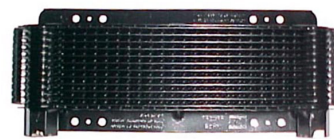
Radiateur d'huile avec 24 plaques 280 x 125 x 40mm
