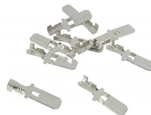
Cosses à sertir plates mâles sans isolation sans barbe, lot de 10 pièces Taille du connecteur: 6,3mm, Épaisseur du matériau: 0,8mm, Épaisseur du fil: 0,5-2,5mm 2
