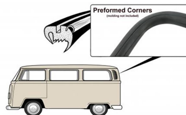
Achterruit rubber deluxe Bus deluxe 8.1967 t/m 7.1971 (behalve Pick-up), gebruik ook #20329
