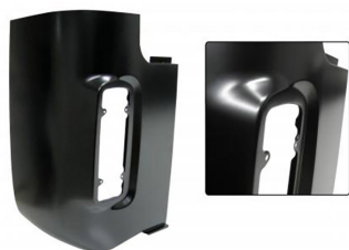
Achterhoek onderzijde links Bus 8.1971 t/m 7.1979 (behalve Pick Up)
