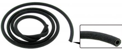
Brandstofslang slang met textiel buitenzijde per meter Binnendiameter: 5.0mm, Buitendiameter: 9.5mm, Working pressure: 7 bar, Bursting pressure: 30 bar
