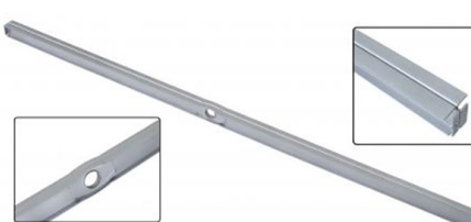
Middelste steunbalk onder de laadvloer (H-profiel) (per stuk) Bus 4.1955 t/m 7.1979
